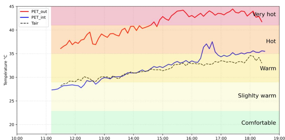
Figure 2 Evolution de la température ressentie en-dehors (rouge) et à l'intérieur (bleu) du Pavillon, ainsi que de la température de l'air (traitillé). Source : demo-mi2@hefr.ch HEIA-FR 2023
